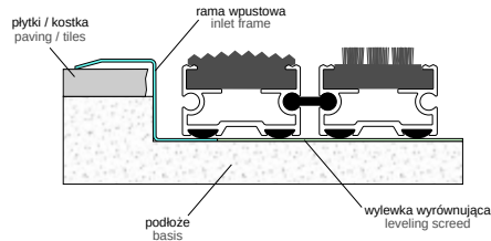
Instalacja z ramą maskującą Installation with masking frame
